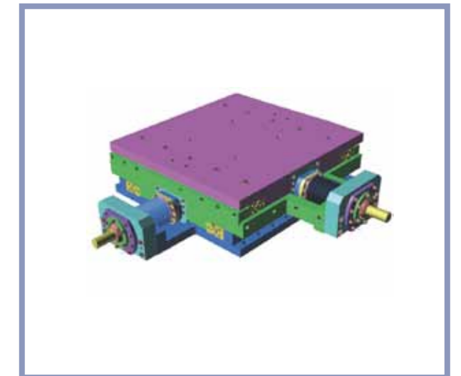
XY 500 Unità a coordinate supporto pezzi per saldatrice componenti acciaio inox. Corsa 200 x 200 mm.
