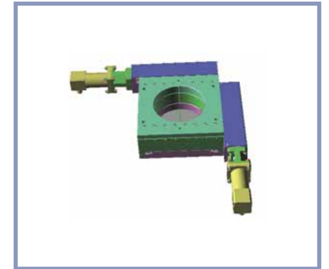
XY 210 Posizionamento dispositivo ottico per laboratorio metallurgia. Corsa 150x150 mm
