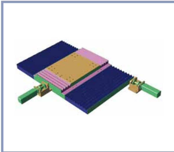
Prototipo Tavola portapezzo per lavorazione con taglio laser. Corsa 600x400 mm
