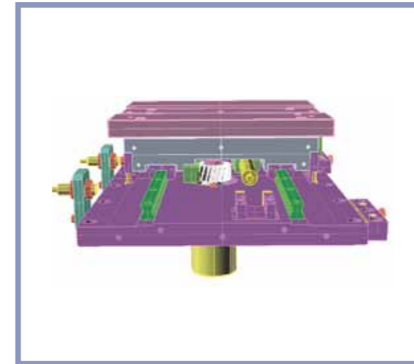
Slitta comando idraulico Posizionamento pezzi su linea transfert. Comando con attuatore idraulico rotativo. Corsa 250 mm
