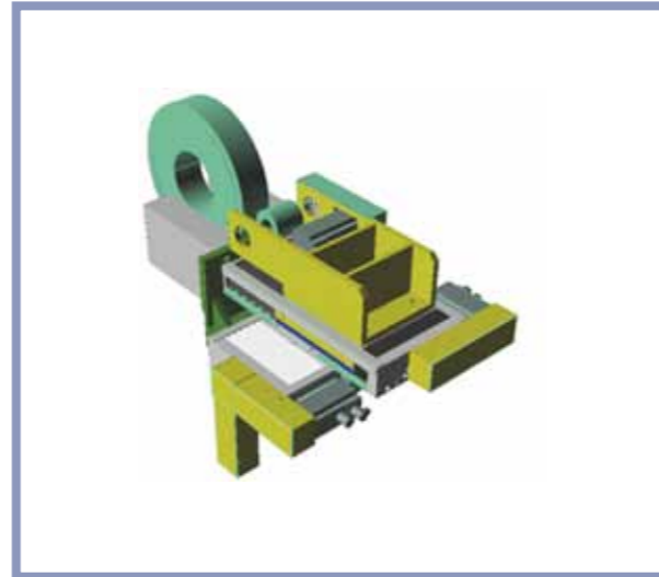
TV4 XY Profilatore mola CNC con elettromandrino integrato per rettificatrice filetti. Corsa 150 x 150 mm
