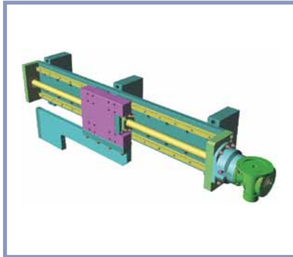
Estrattore bobine Asservimento macchina lavorazione gomma. Comando con vite e motoriduttore. Corsa 600 m
